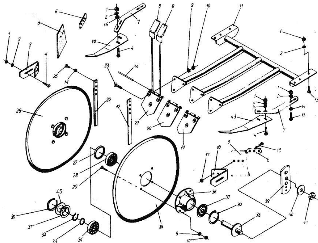
Rys. Do tablicy T-8. Lemiesz z kręgiem środkowym
